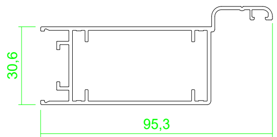
Rahmenprofil mit Schlagleiste 000173
