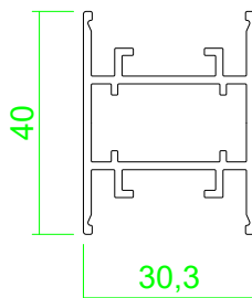
Sprossenprofil (klein)
