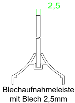
Blechaufnahmeleiste
