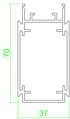
Rahmenprofil
