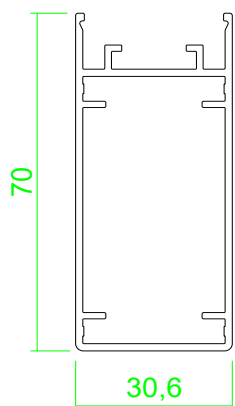
Rahmenprofil
