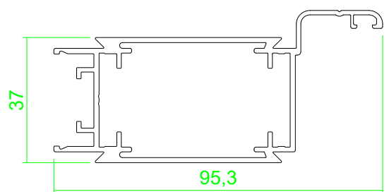
Rahmenprofil mit Schlagleiste
