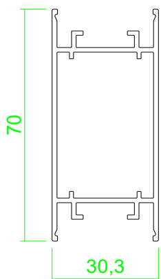
Sprossenprofil
