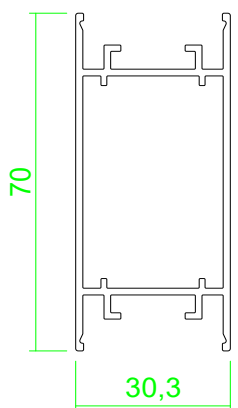
Sprossenprofil
