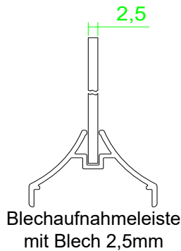
Blechaufnahmeleiste
