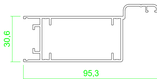
Rahmenprofil mit Schlagleiste
