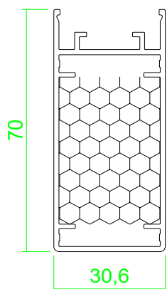
Rahmenprofil 000184
