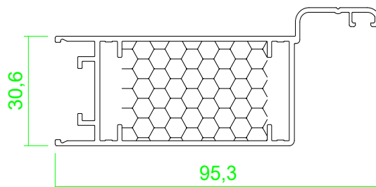
Rahmenprofil mit Schlagleiste 000173 i
